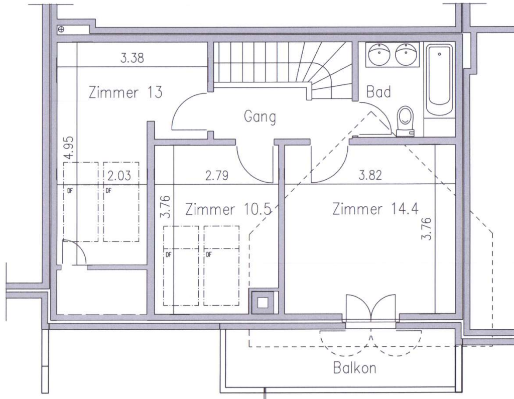
Grundriss Dachgeschoss 4 1/2 – Maisonnette-Wohnung Nr. 2
