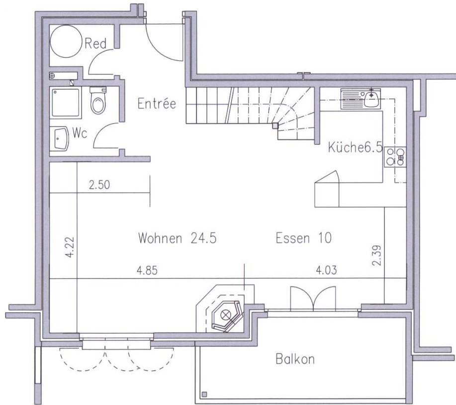
Grundriss Obergeschoss 4 1/2 – Maisonnette-Wohnung Nr. 2
