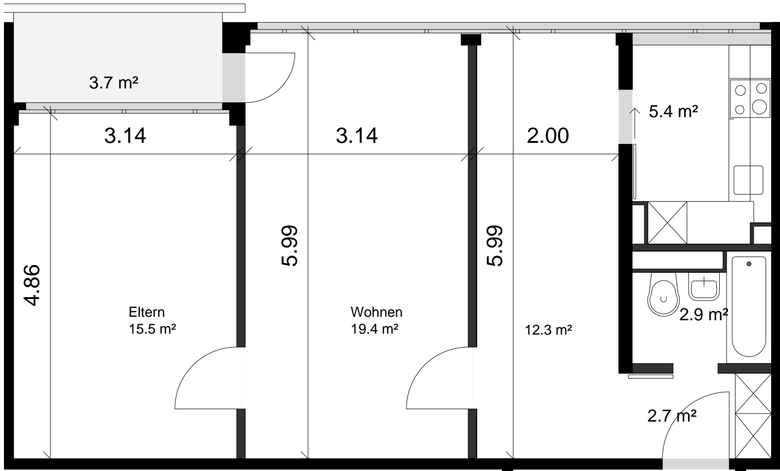
Grundrissplan
