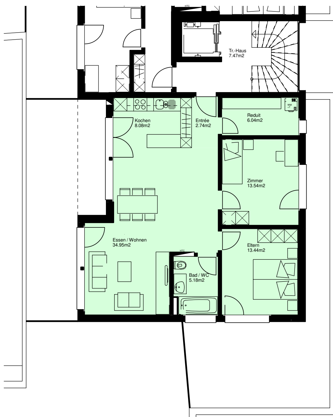
Grundrissausschnitt Attikageschoss 64 3½ Zimmerwohnung
