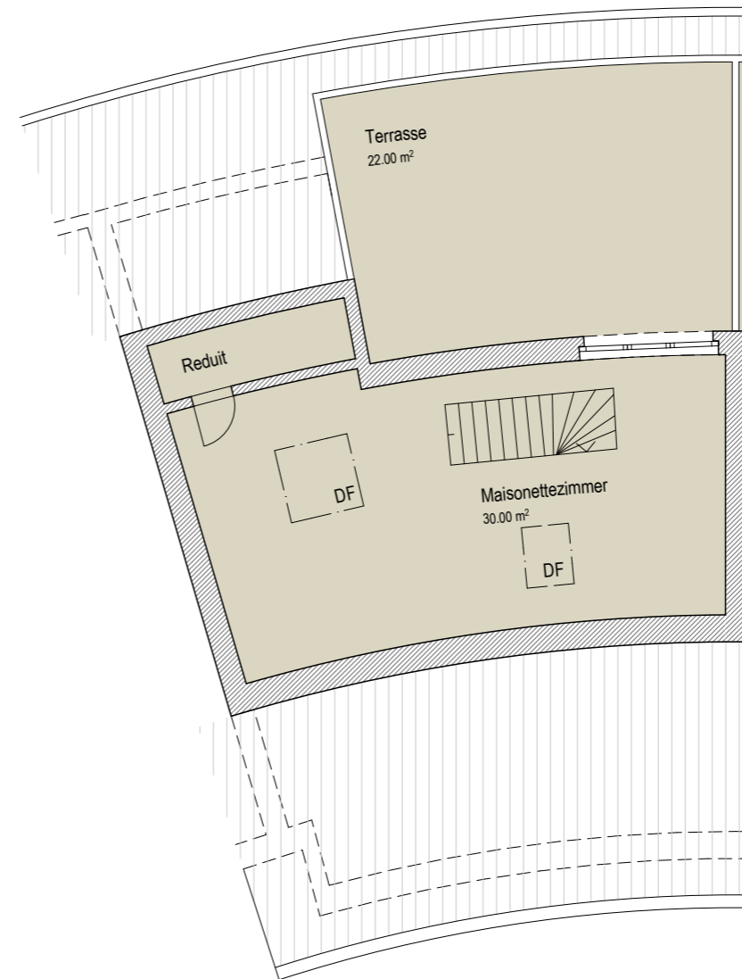
Dachgeschoss
