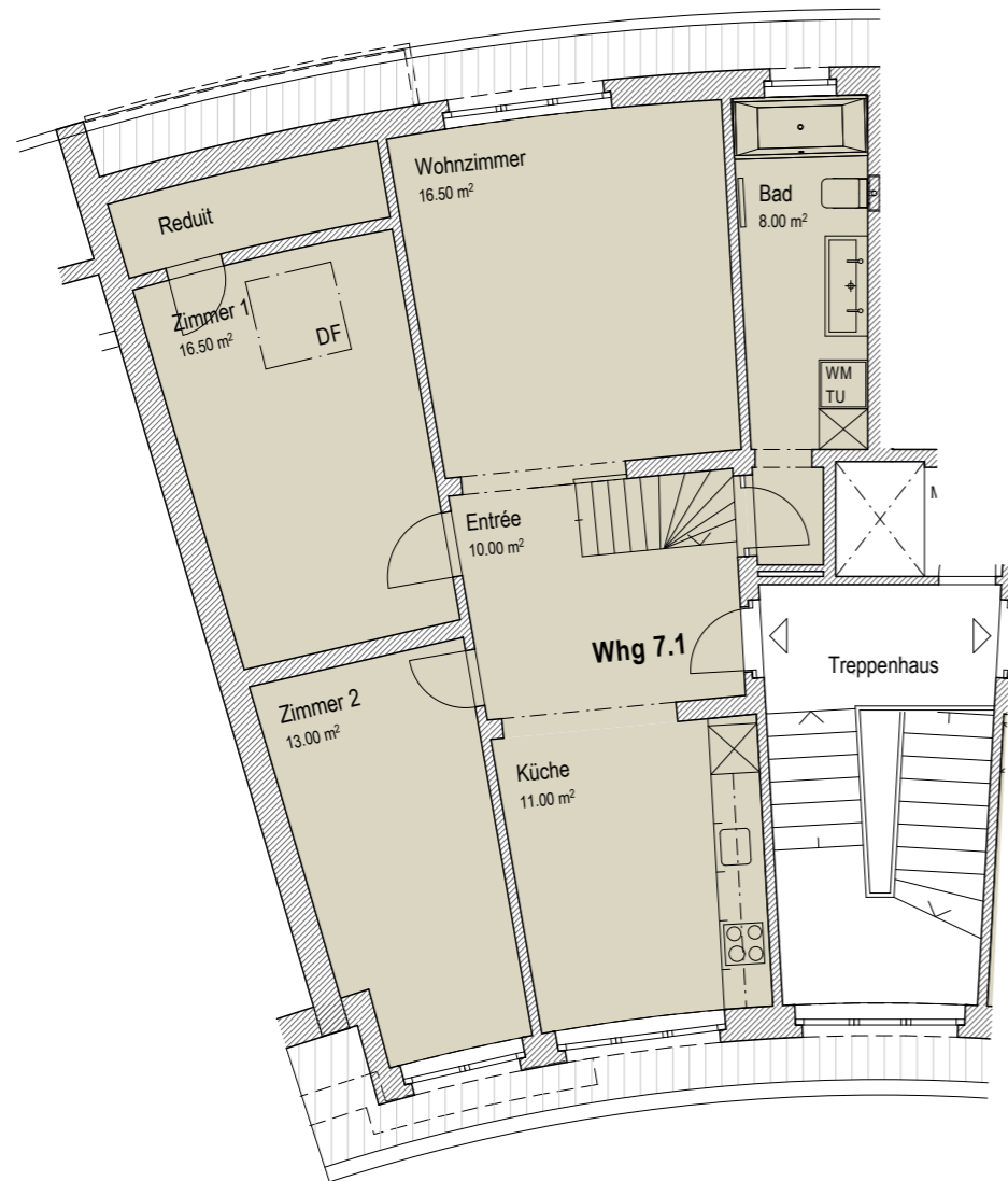
6. Obergeschoss
