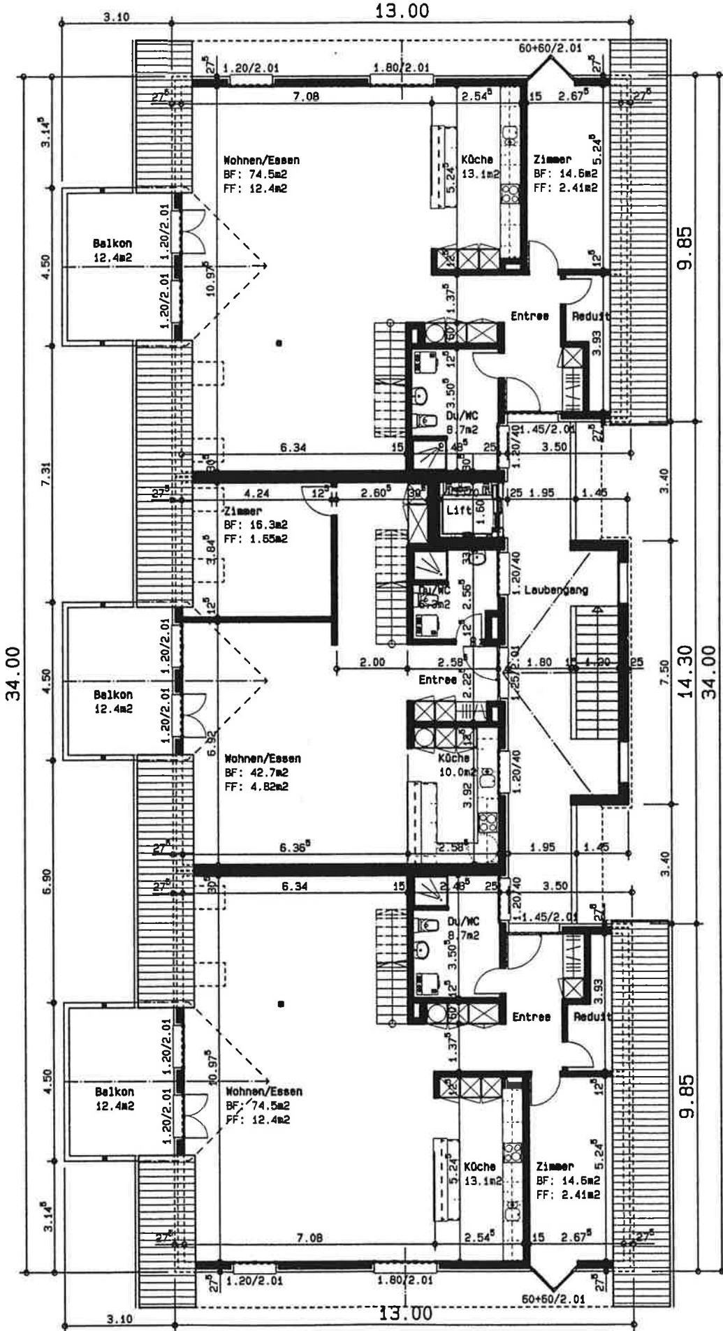
Grundriss Dachgeschoss ( Haus H ) Mst. 1:150
