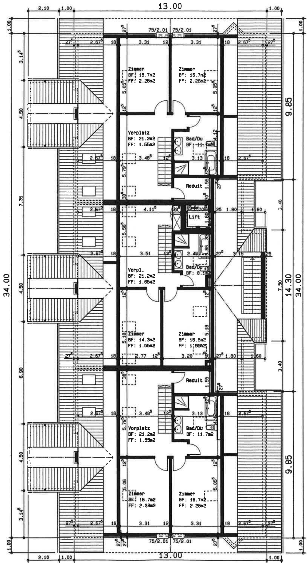
Grundriss Galerie ( Haus H ) Mst. 1:150
