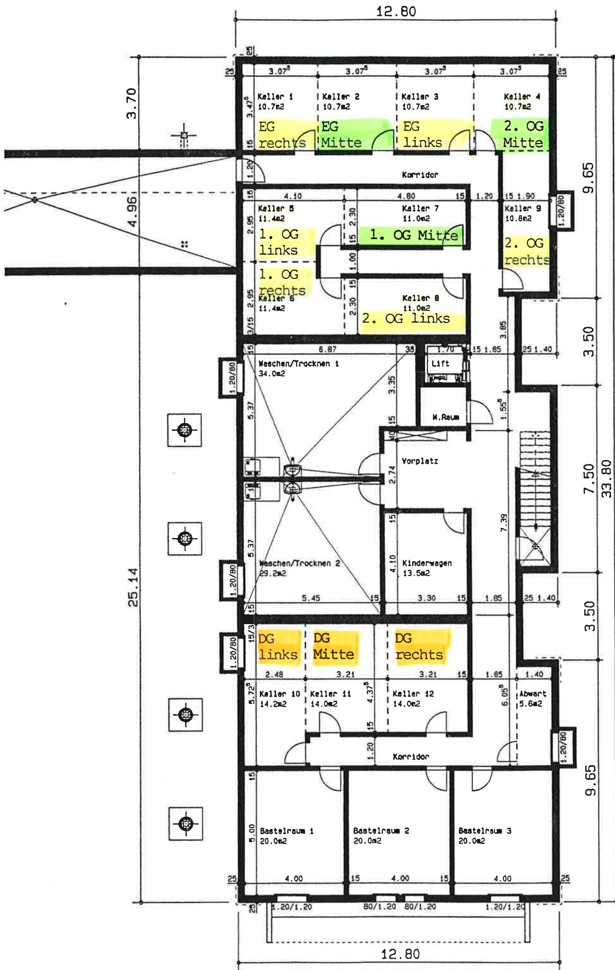
Grundriss Untergeschoss ( Haus H ) Mst. 1:150
