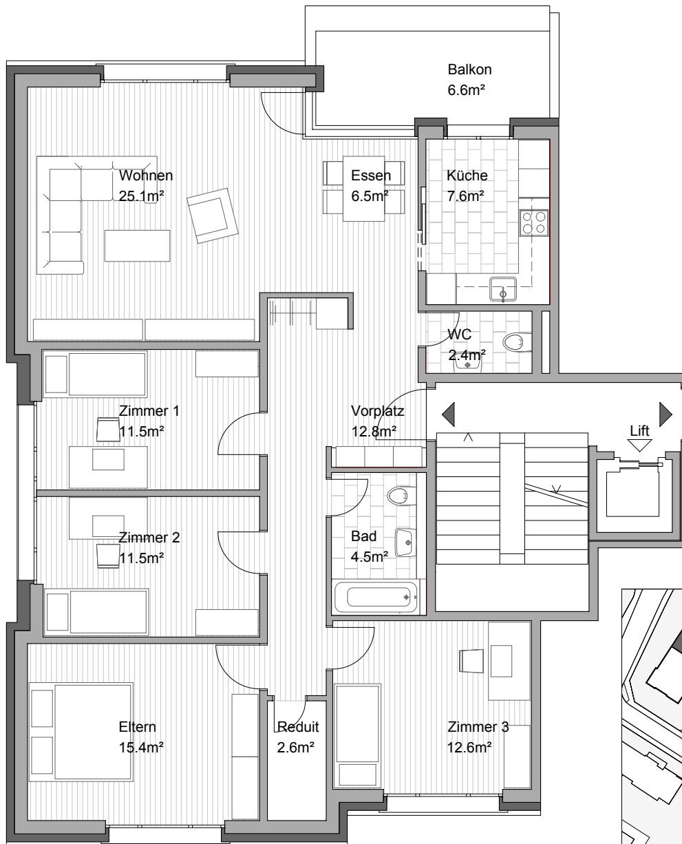
Grundriss MST. 1:100
