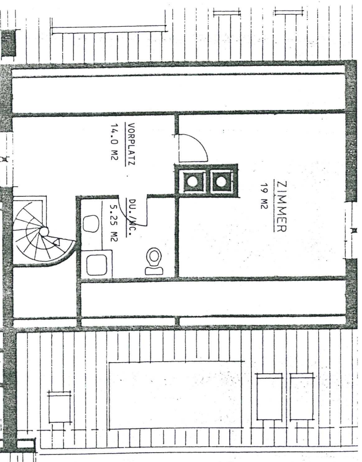
GRUNDRISS DG.
