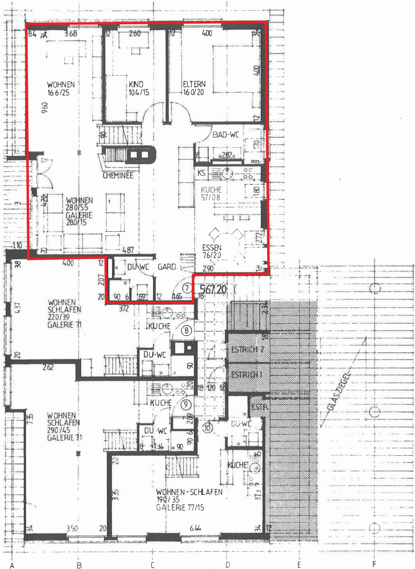
GRUNDRISS DACHGESCHOSS
