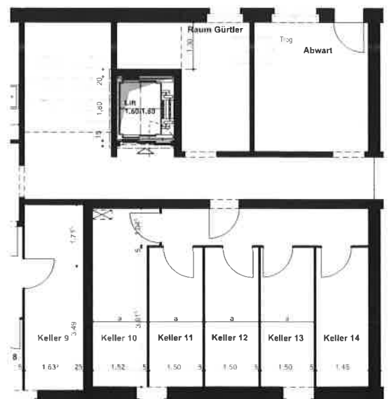
Grundriss Kellerabteile Untergeschoss Massstab 1:100
