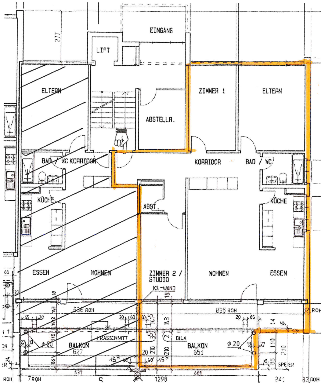
Grundrissplan / Begründungsplan 4 1/2 - Zimmerwohnung (nicht massstäblich)
