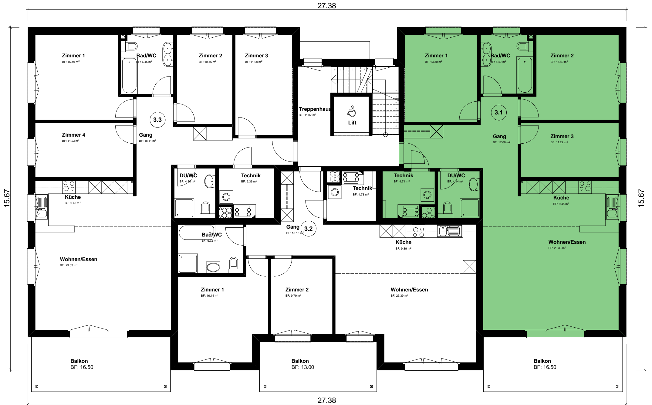
2.OBERGESCHOSS HAUS A/B/C/E/F
