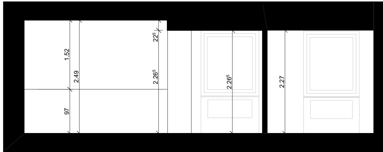
Schnitt B
