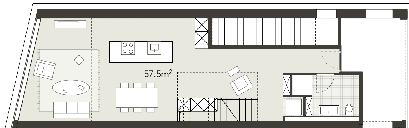
Zugangsgeschoss (1.OG)
